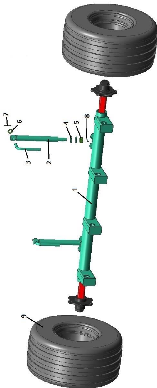
Ось колес КПМ-16 21.080 в сборе с винтами
