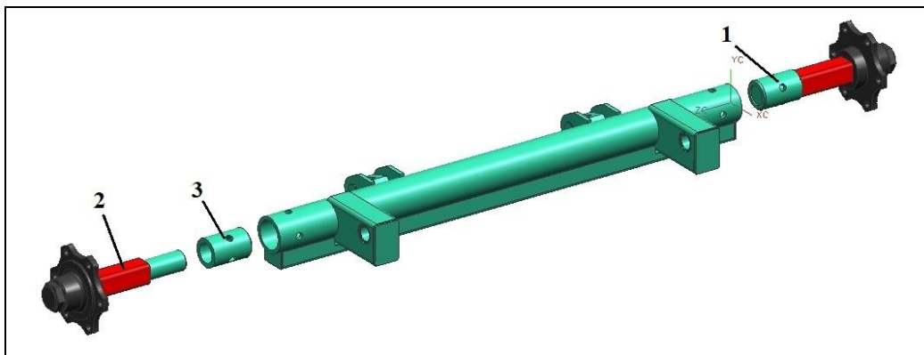
КПМ-12-У 01.180Д Ось колес (Сварной узел)
