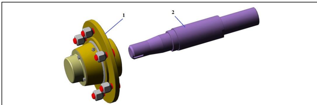
КПМ-10 05.090 Полуось
