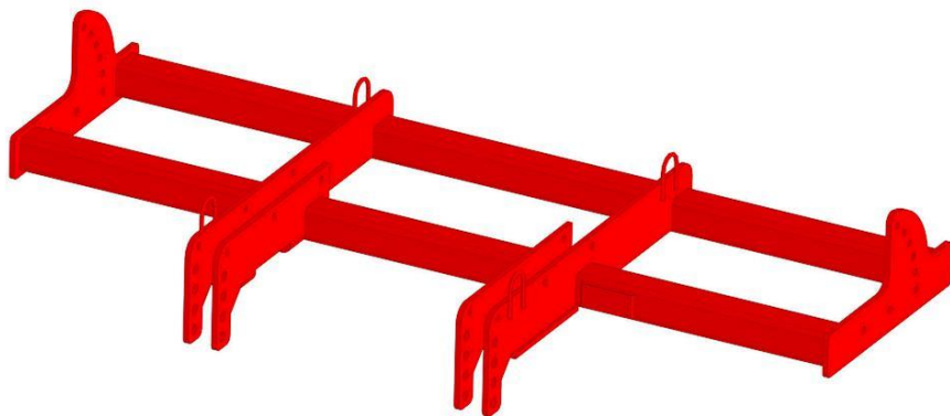
ГРШ 01.010 Рама КГР-1,6 01.000 Рама КГР-3,2 01.000 Рама
