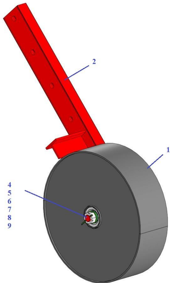
ГРШ 03.000 Колесо копирующее
