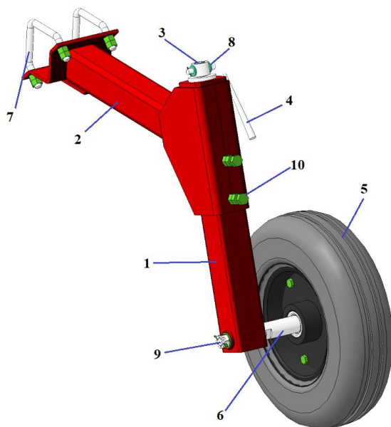
КГО 05.040 Колесо опорное
