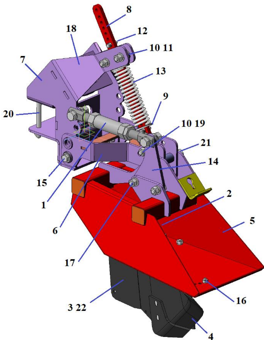
КГО 14.020-02 Полоз правый в сборе
