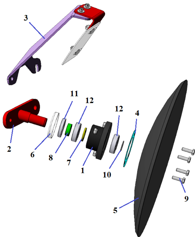
КГО 10.600 Р-01 Ось в сборе
