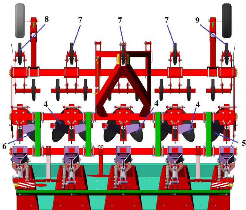
КУЛЬТИВАТОРЫ-ГРЕБНЕОБРАЗОВАТЕЛИ КГО-2,8 / КГО-3,0 / КГО-3,6 Общий вид
