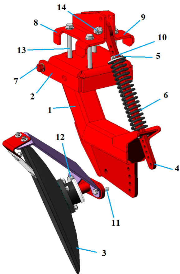
КГО 10.000 У-02 Окучник дисковый
