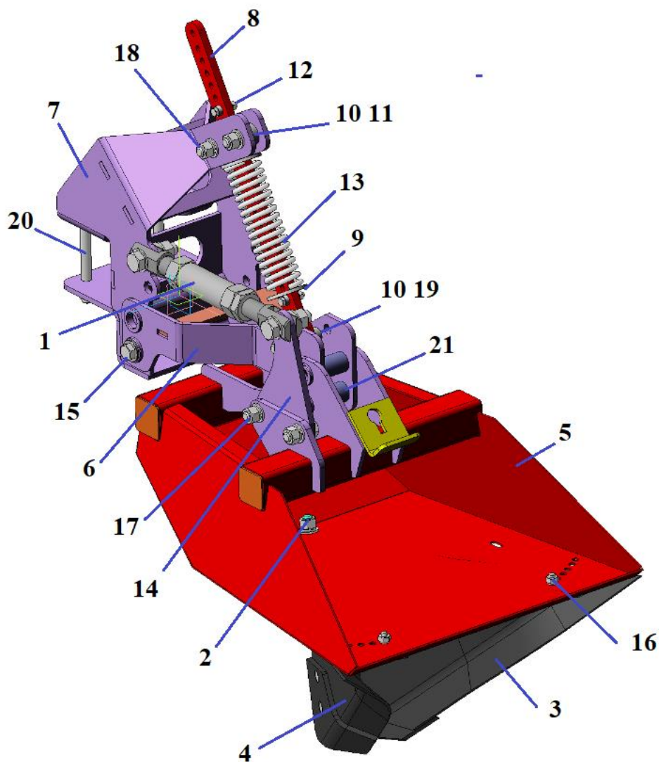
КГО 14.020 Полоз средний в сборе
