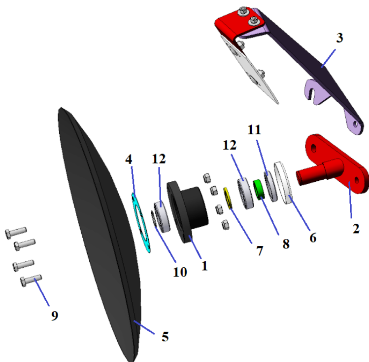
КГО 10.600 Р Ось в сборе
