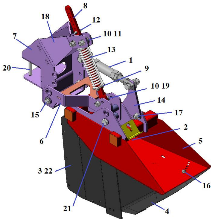
КГО 14.020-01 Полоз левый в сборе
