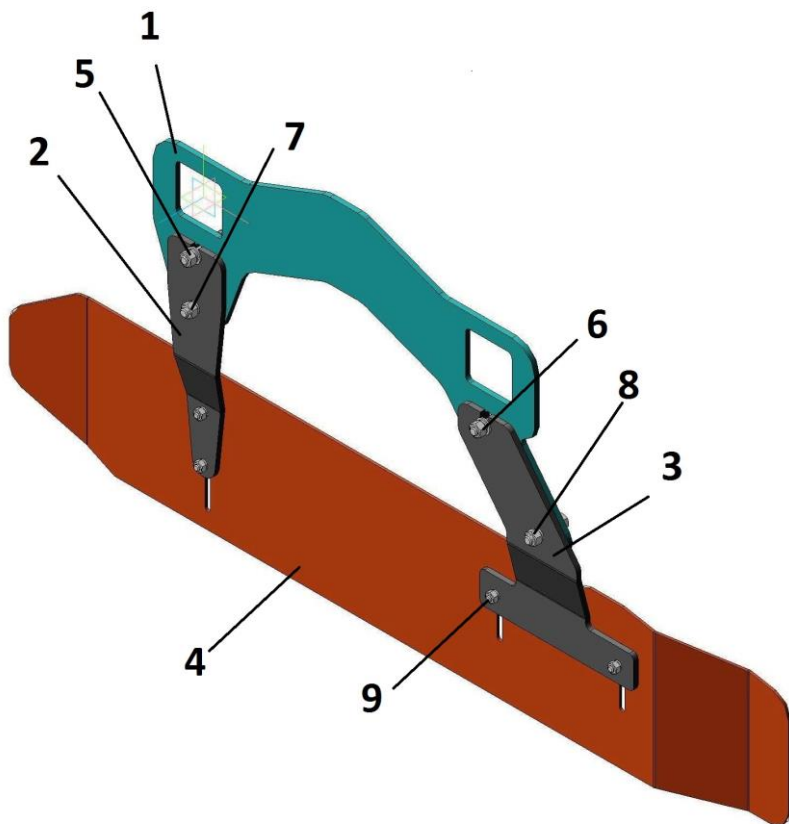
КГО 12.030 А Ограждение
