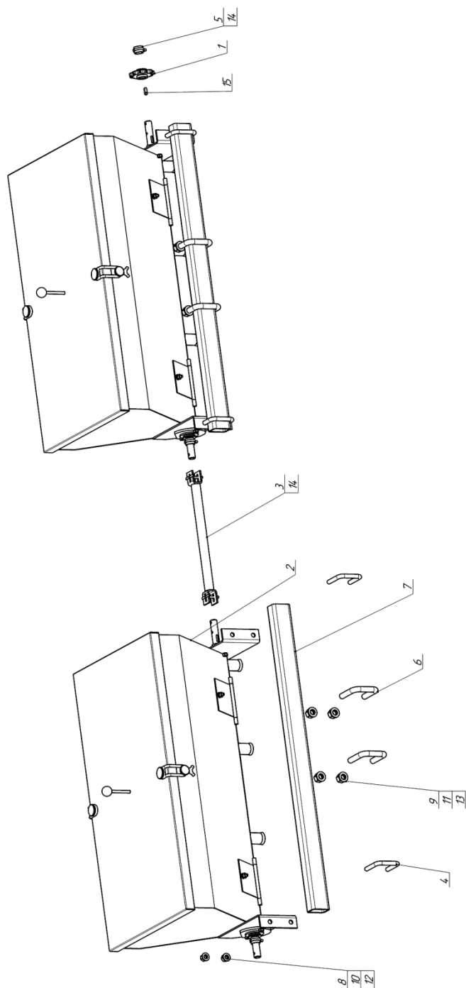
СПК 02.000 А Аппарат туковывевающий
