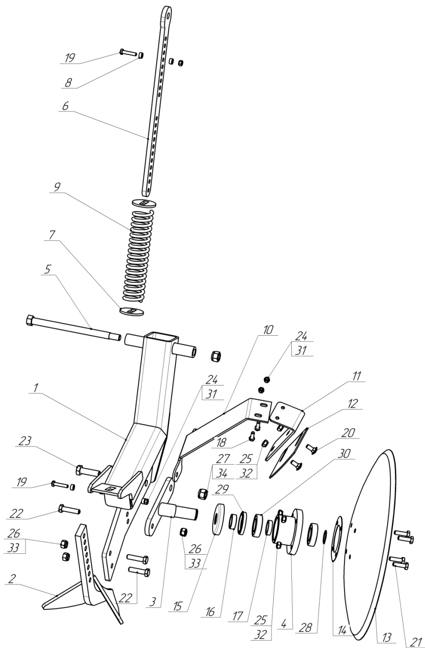
СПК 07.200 Окучник дисковый левый
