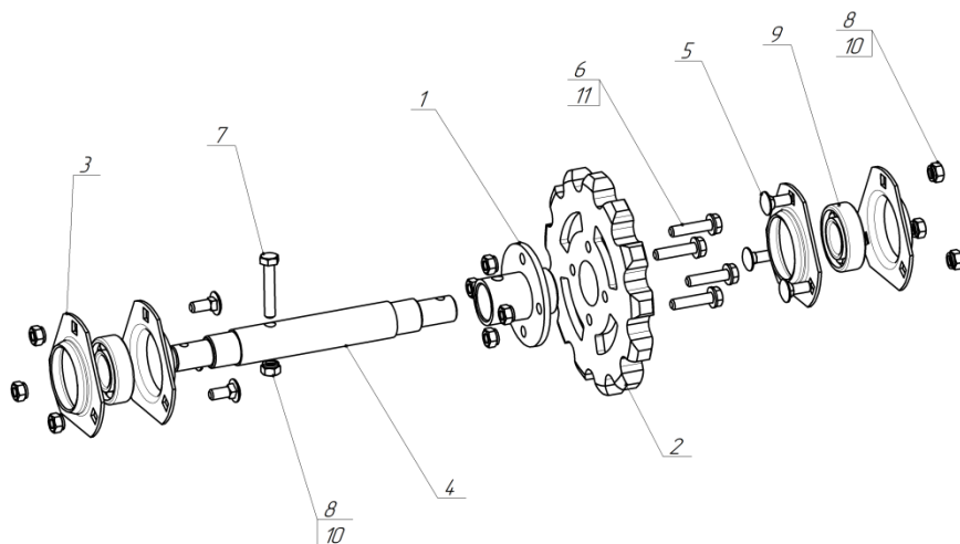
СПК 05.450 Вал нижний
