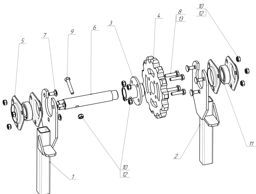
СПК 05.440 Механизм приводной верхний
