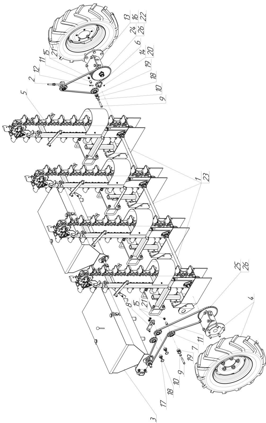
Привод СПК-4-70
