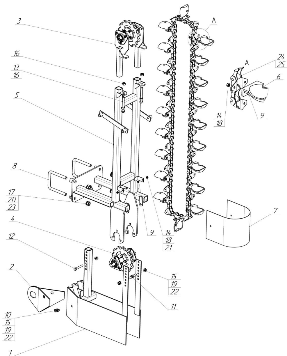
СПК 05.000 А Механизм высаживающий
