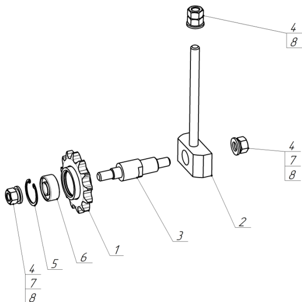
СПК 00.210 Звездочка натяжная
