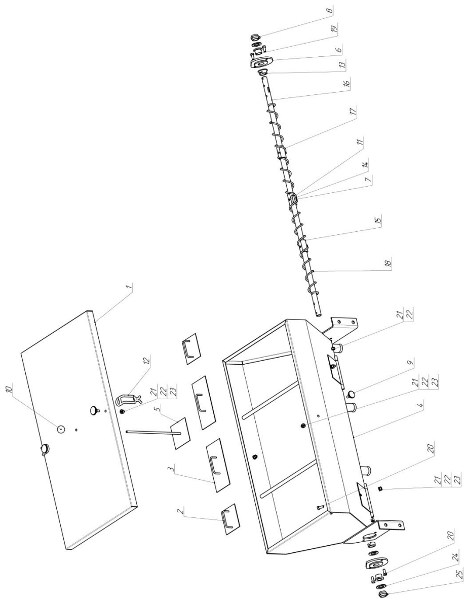
СПК 02.150 А Бункер в сборе
