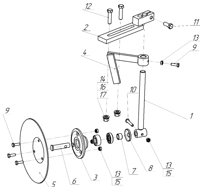
СЛ 04.26.000 А Загортач
