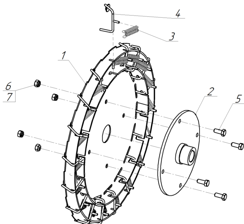
СЛ 03.00.000 Аппарат высаживающий
