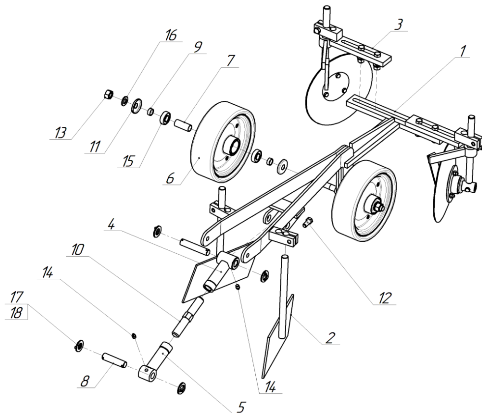
СЛ 04.15.000 Колёса прикатывающие
