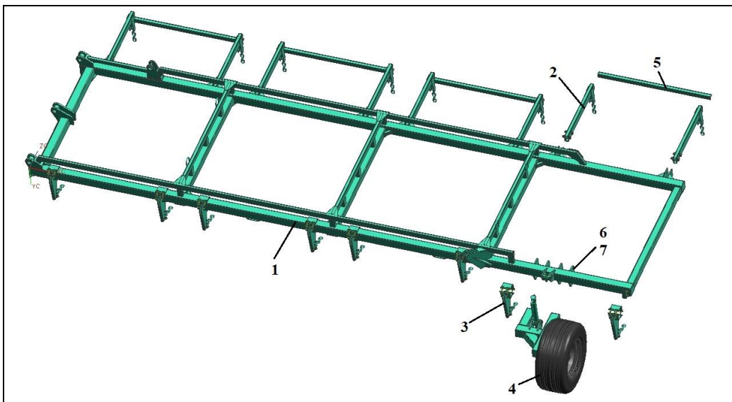
БЗС-22 03.000 А-01 Крыло левое
