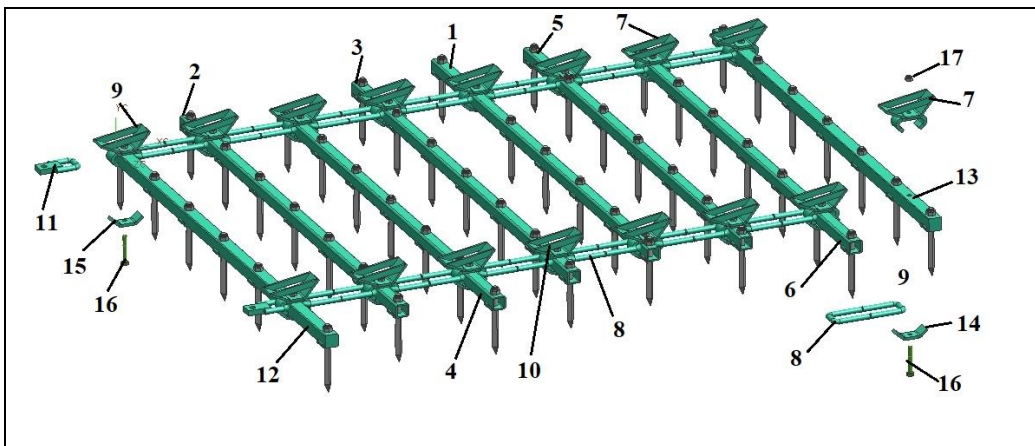
БЗС-18 06.010 Л Полуполотно
