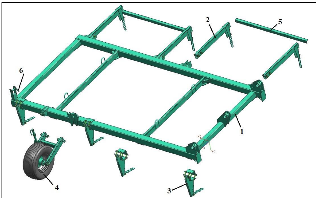
БЗС-22 04.000 А Открылок правый
