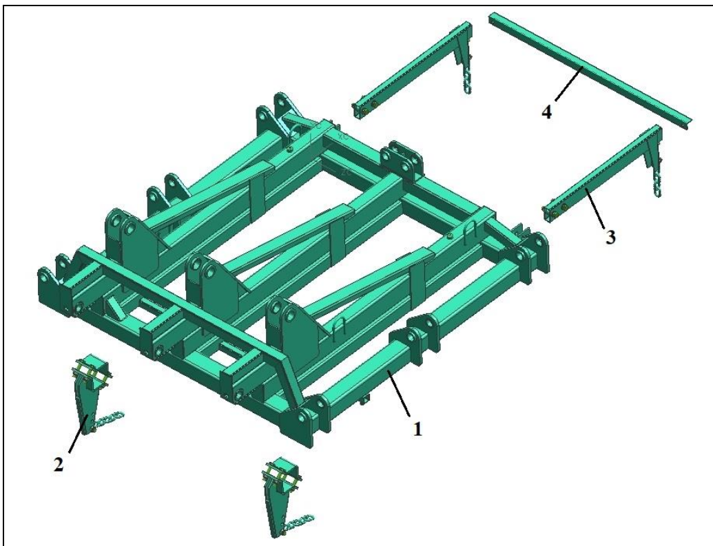
БЗС-22 02.000 Секция центральная
