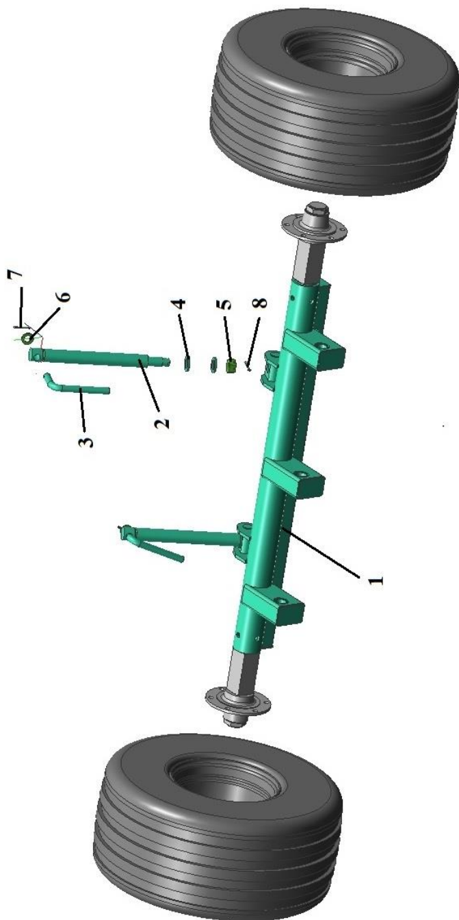
Ось ходовых колес БЗС-22 01.080 в сборе с винтами
