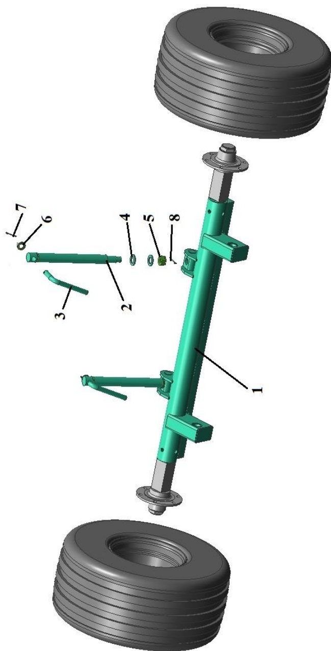
Ось ходовых колес БЗС-15 21.080 в сборе с винтами
