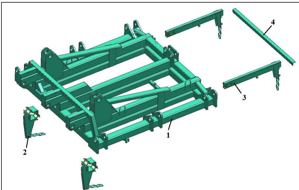
БЗС-15 22.000 Секция центральная
