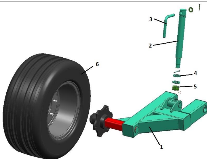
БЗС-22 03.150 Колесо для разворота (правое) БЗС-22 03.150-01 Колесо для разворота (левое)
