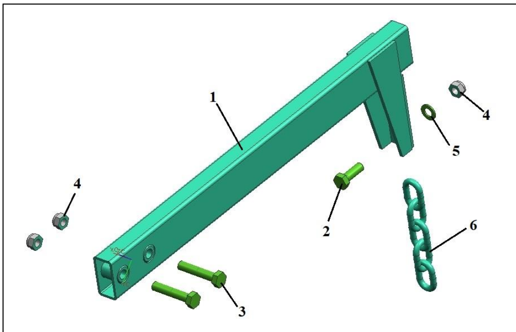
БЗС-22 05.060 Кронштейн задний
