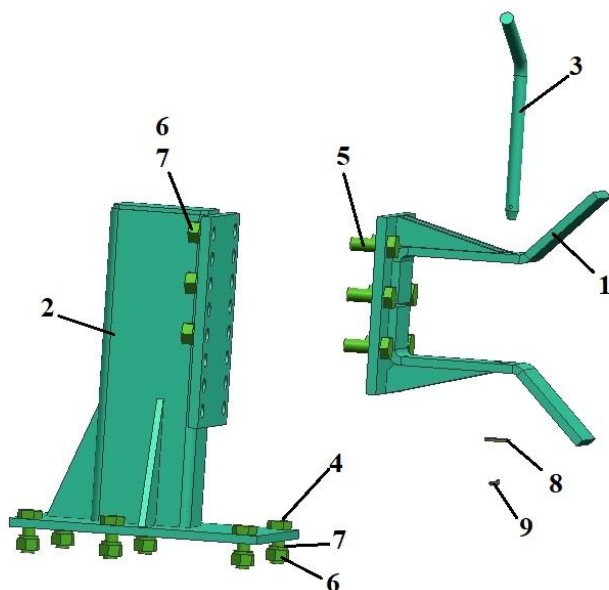
БЗС-11,5 01.150 Ловитель
