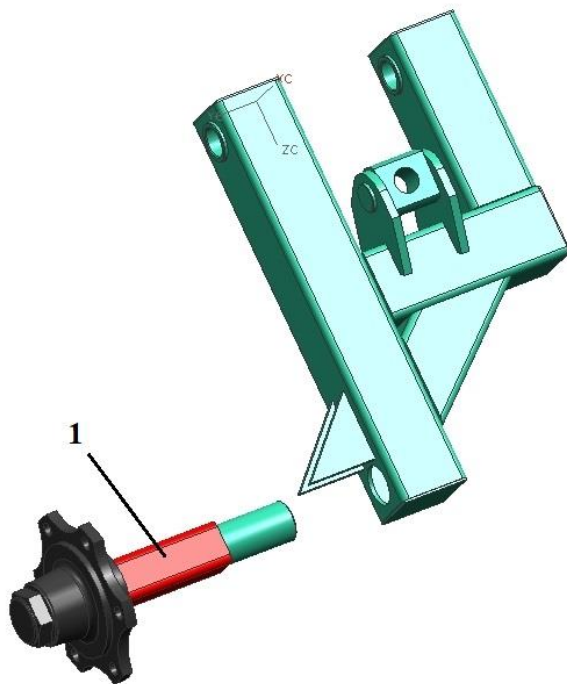
БЗС-22 03.160 Кронштейн колеса БЗС-22 03.160-01 Кронштейн колеса (Сварные узлы)
