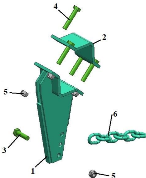
БЗС-11 05.040 Д Кронштейн передний
