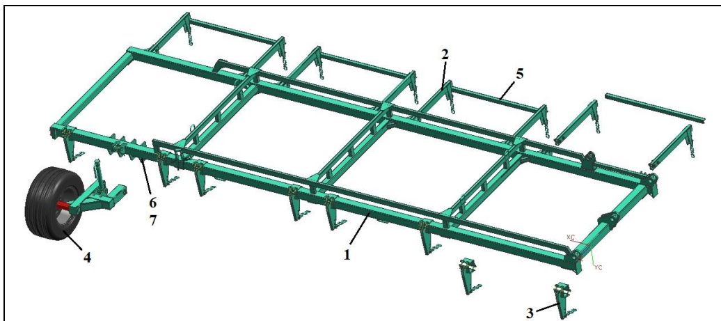
БЗС-15 23.000 А Крыло правое
