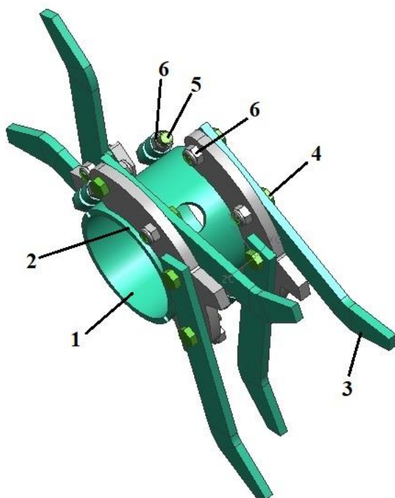
АПК-75Н 03.100 Н-01 Полувставка средняя
