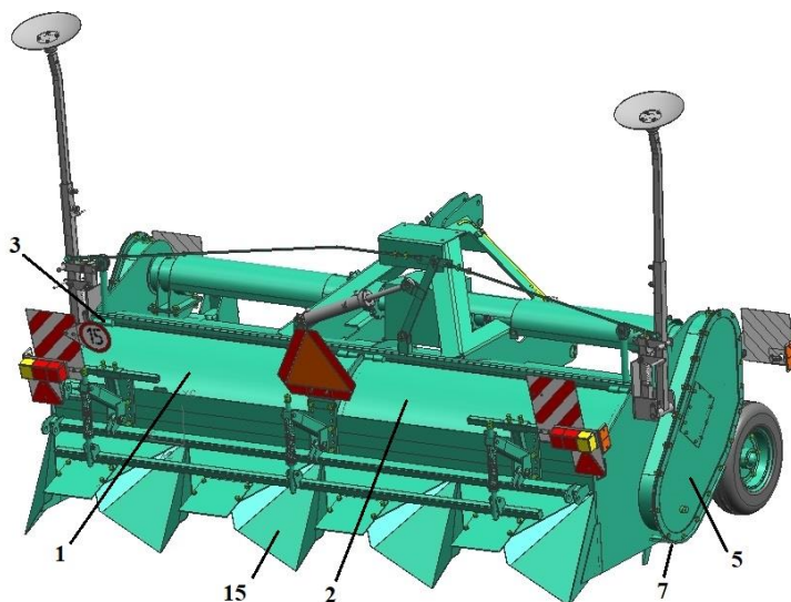
АПК-3,0 Общий вид
