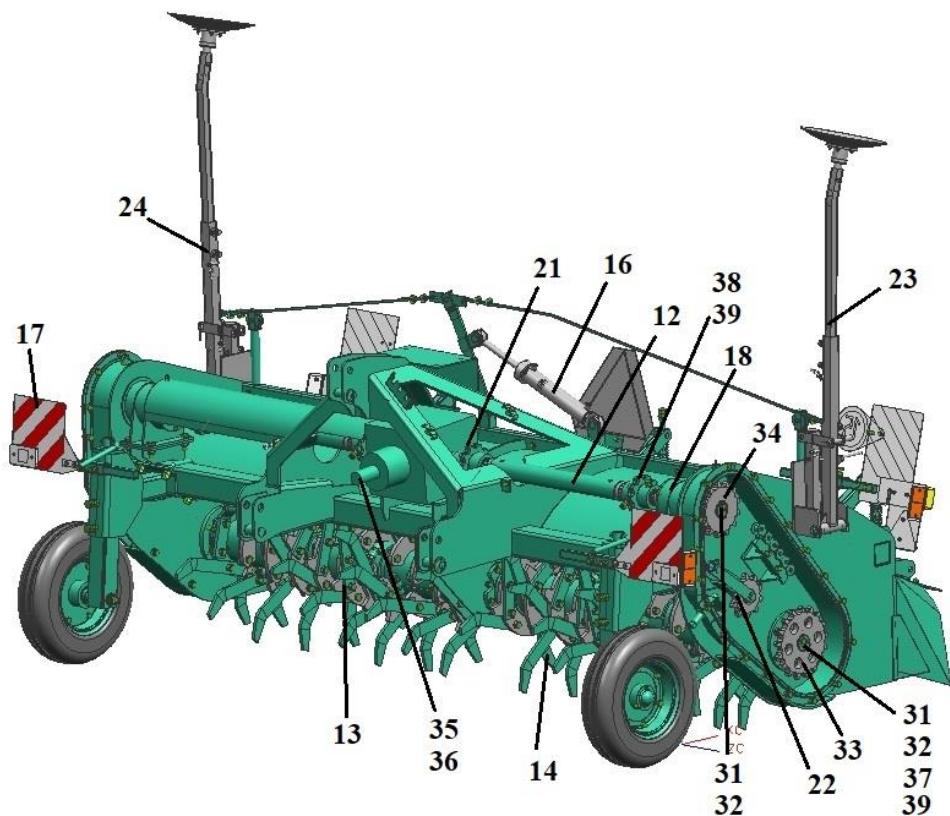
АПК-3,0 Общий вид
