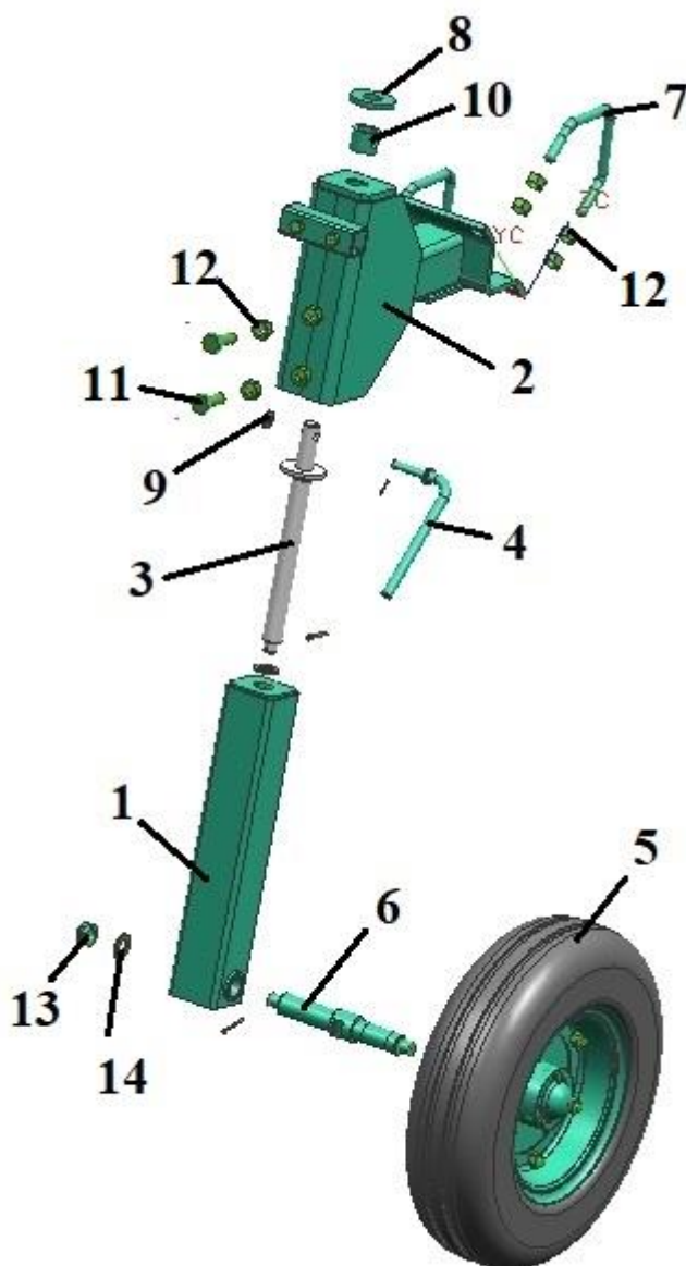
АПК-1,4 05.040 Д Колесо опорное / АПК-1,4 05.040 Д-01 Колесо опорное
