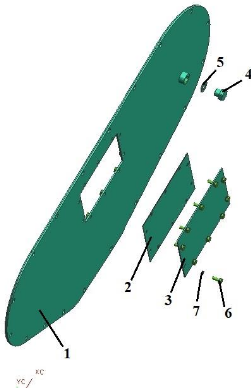
АПК-70 00.090 В Крышка корпуса левая / *АПК-70 00.090 В-01 Крышка корпуса правая
