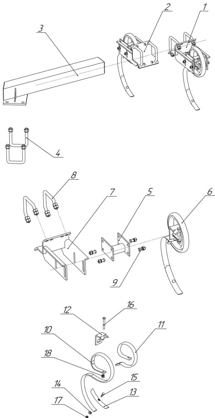
АКШ 01.04.000А Следорыхлитель АКШ 01.04.000А-01 Следорыхлитель (зеркально)
