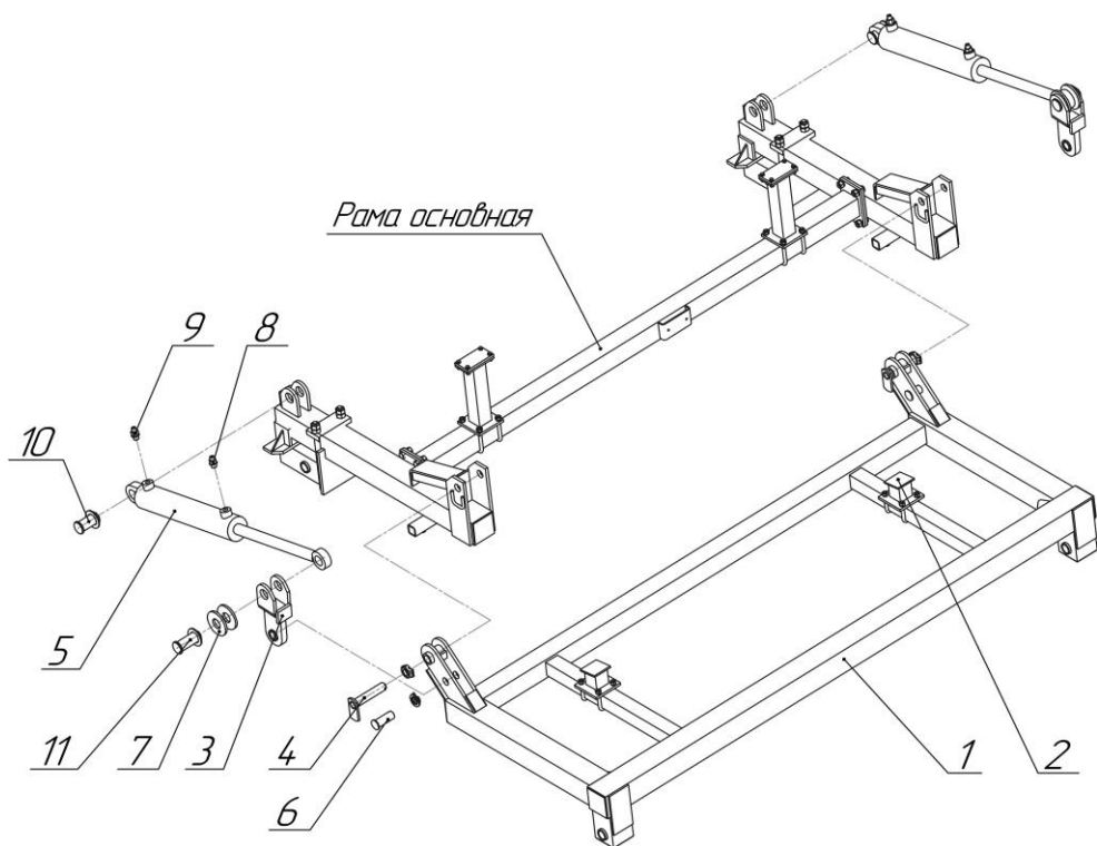
АКШ 73.00.000 Рама боковая (с креплением)
