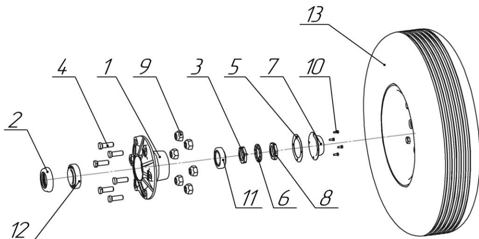
Колесо 8,25-15 Колесо со ступицей
