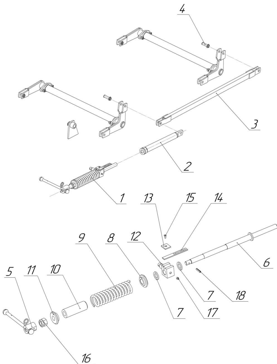
Устройство демпфирующее
