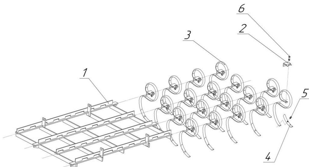
АКШ 02.02.000-02 Рамка
