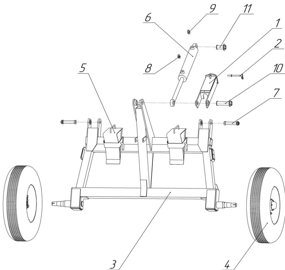
АКШ 64.00.100 Ход колесный (с цилиндром поднятия)
