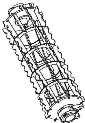
AKШ 62.07.000П-01 Каток
