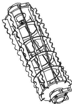
AKШ 62.07.000П Каток
