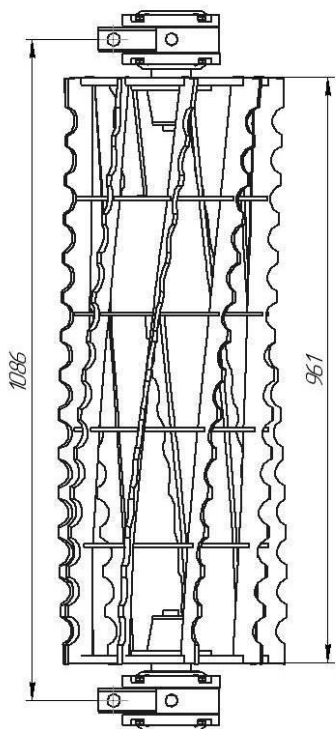
AKШ 62.07.000П Каток
