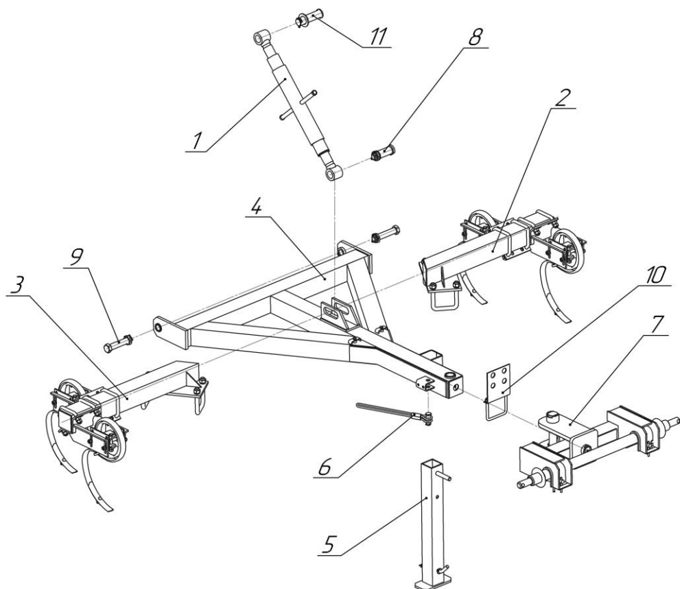
АКШ 65.00.000 Сница (с талрепом регулировки)
