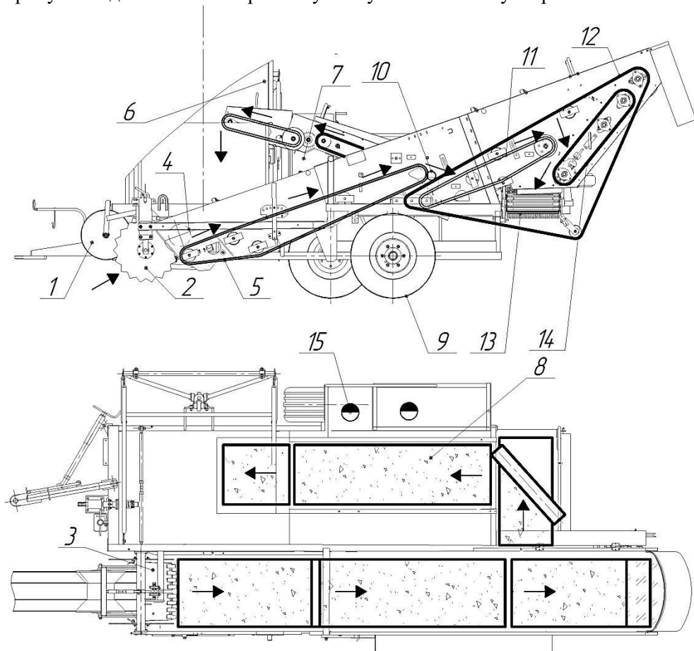
Рисунок 2 – Схема работы комбайна
