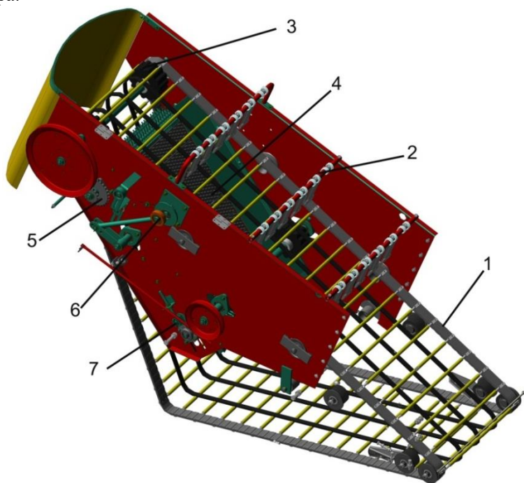
Рисунок 5 – Ботвоудаляющая часть
