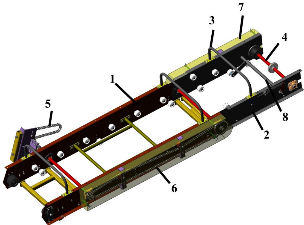
Рисунок 7 – Транспортёр загрузки бункера
