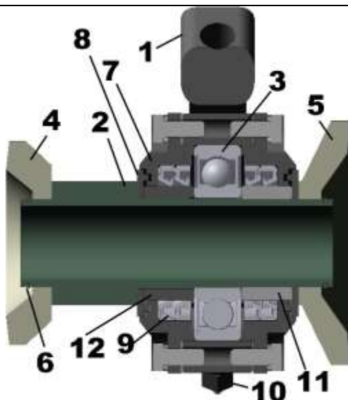
Рисунок 3 – Корпус подшипника
