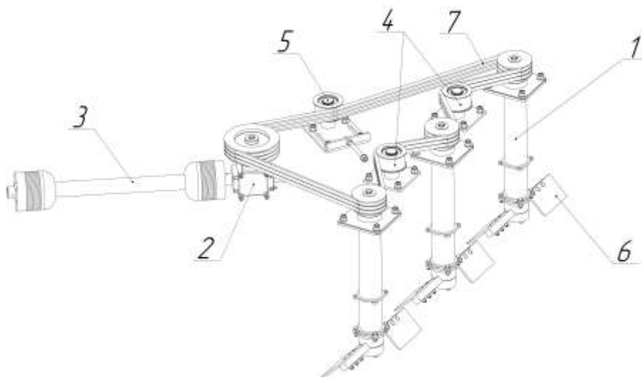
Рисунок 3 – Привод
