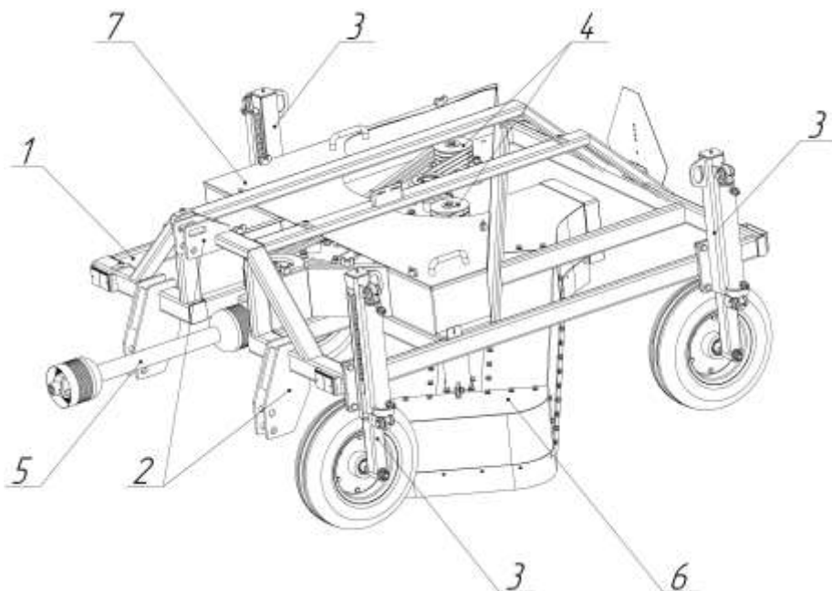
Рисунок 1 – Общий вид машины ботвоуборочной МБУ-1,4ЛК
