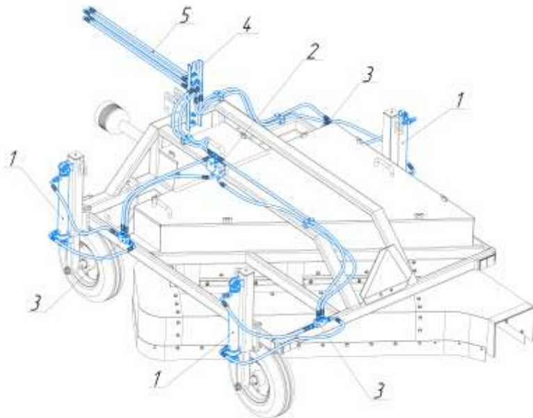
Рисунок 5 – Гидросистема МБУ-1,4ЛК
