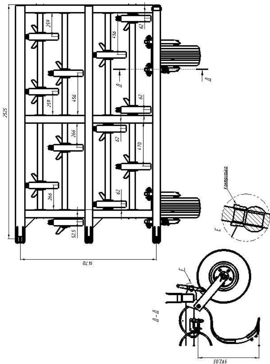
Рисунок 28 – Схема расстановки сток 70x12 левого открыва КПМ-16 (4-х рядный)
