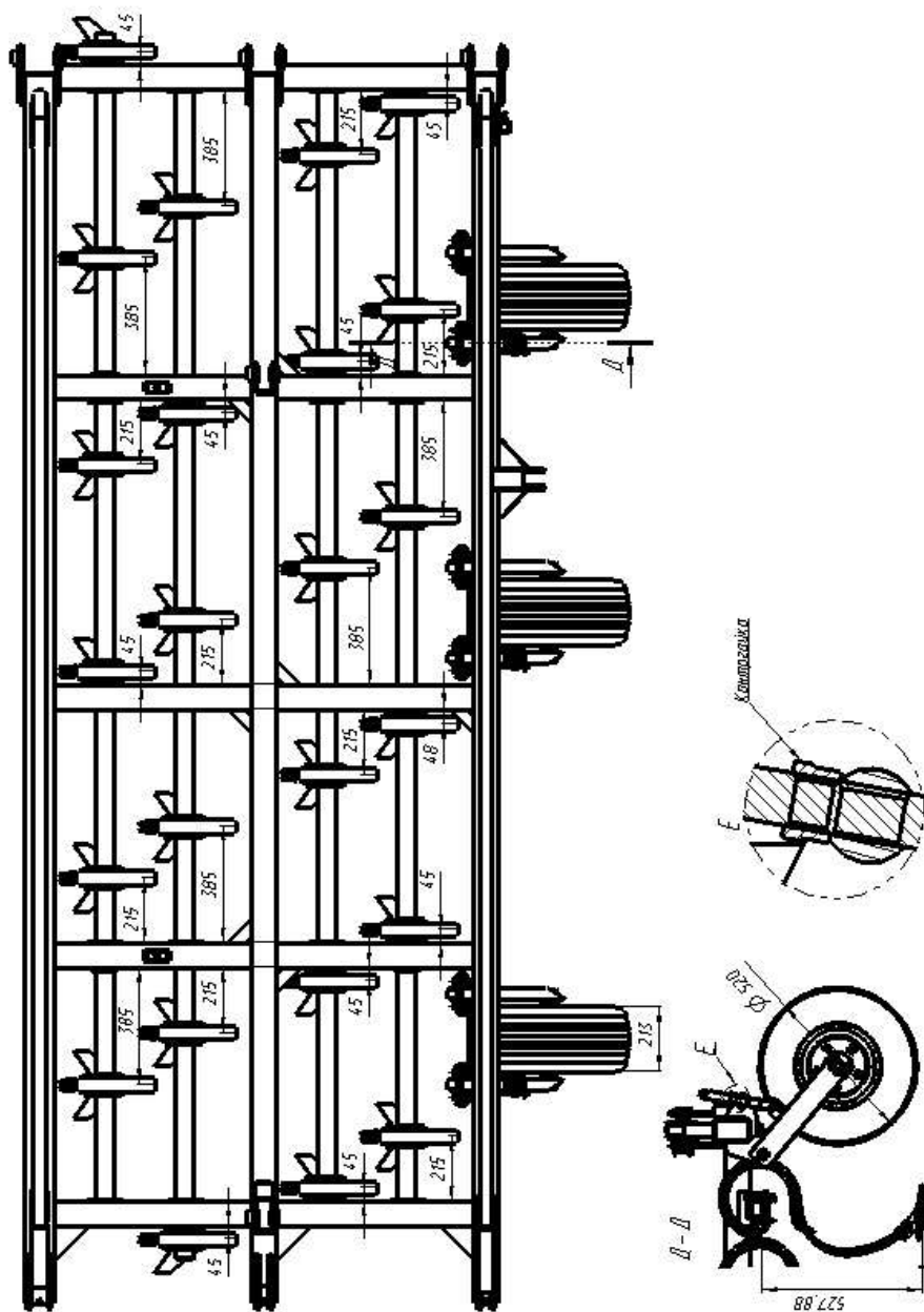
Рисунок 18 – Схема расстановки стоек 45х12 левого крыла КПМ-14 и КПМ-16 (4-х рядных)
